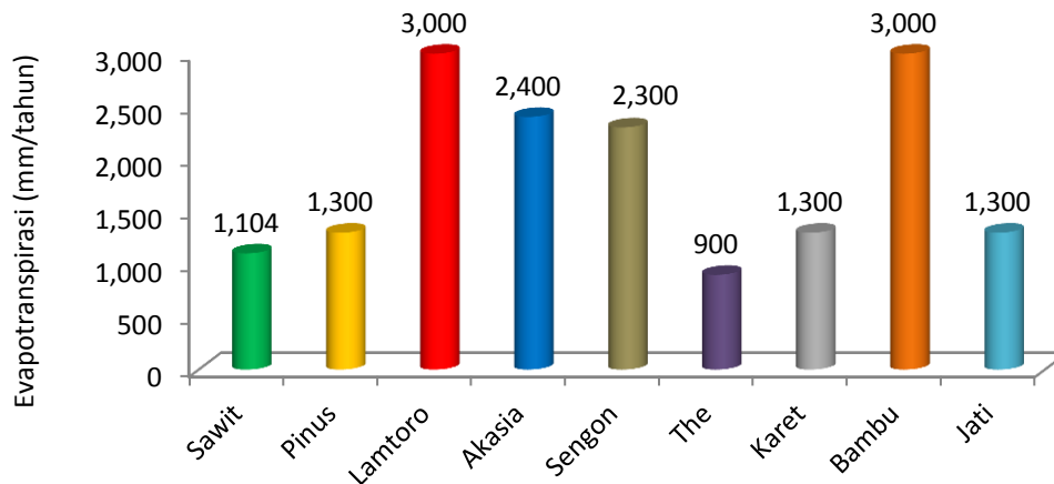
Gambar 2. Perbandingan Kebutuhan Air Kelapa sawit dan Tanaman Hutan (Sumber: Coster, 1938)
